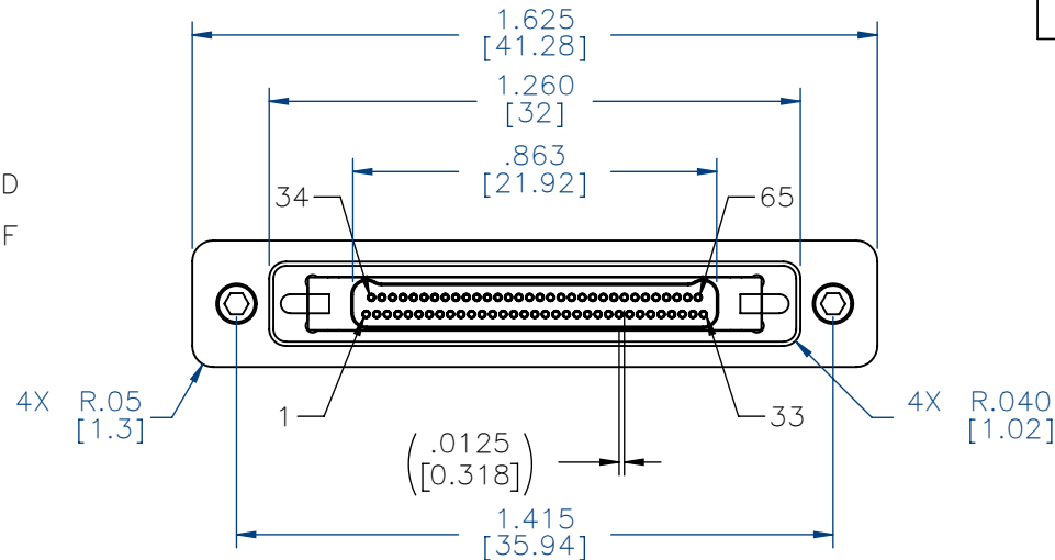
ACTUAL SIZE EXCLUDING WIRE LENGTH
